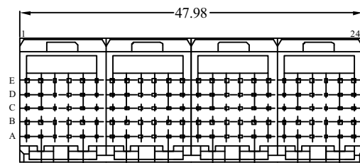
4 Module 89055-113LF
