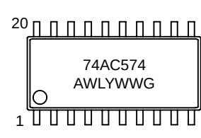
SOEIAJ–20
