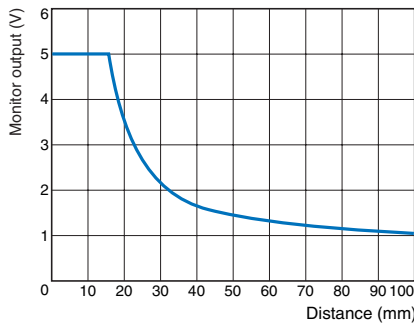
Reflective E32-DC200
