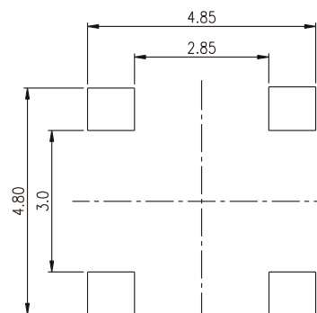
P.C.B. LAYOUT
