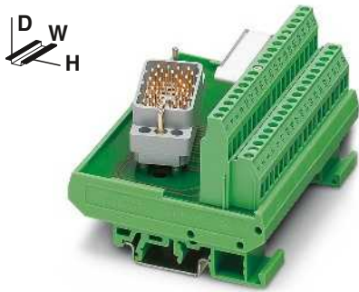
38-pos.
