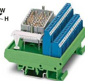
32-pos.
