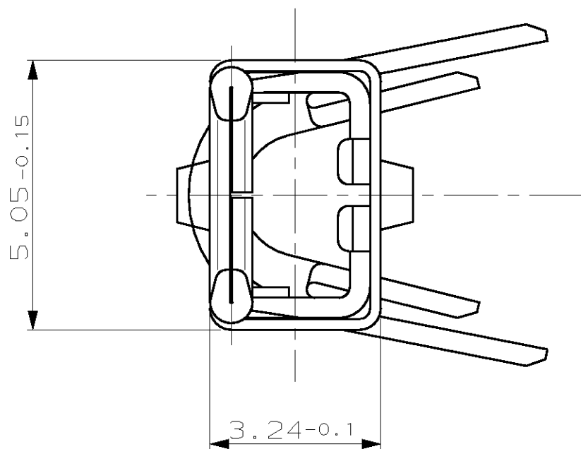
ANSICHT X
