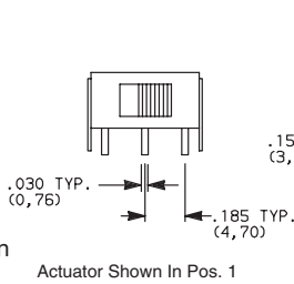
1101M2S3ABE2 Horizontal Actuation SPDT
