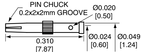
SOCKET
