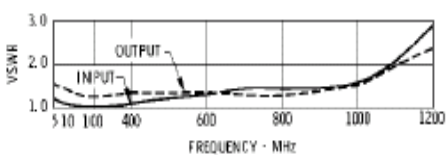
VSWR
