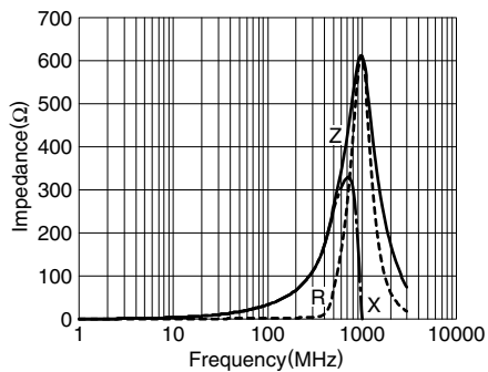
MMZ1005F330C
