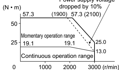
R88M-K4K020(H/T)-□ (4 kW)
