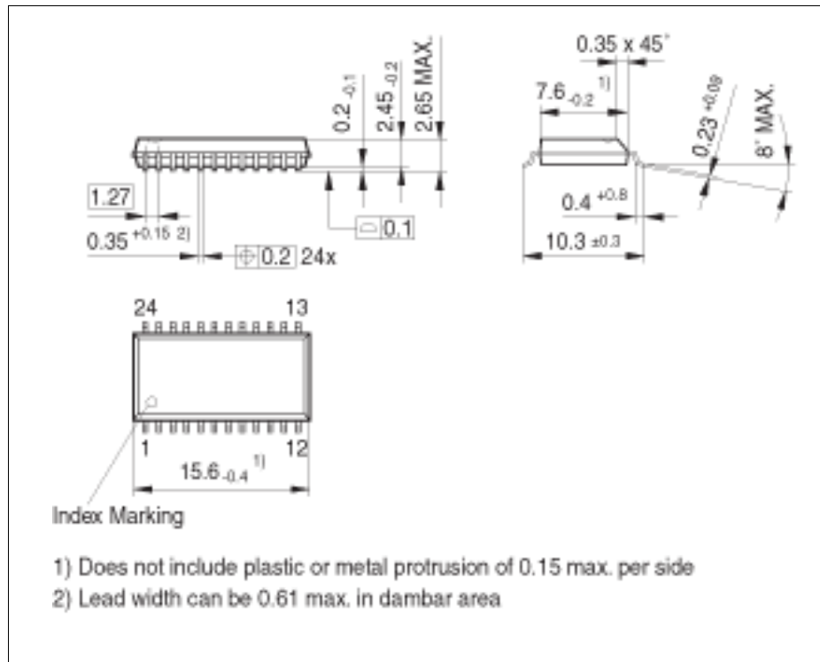
图 17 PG-DSO-24-1 封装图
