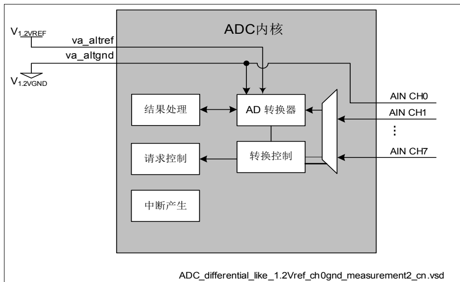
图 9 类差分测量, 使用内部 1.2\text{ V} 电压参考和 CH0 地
