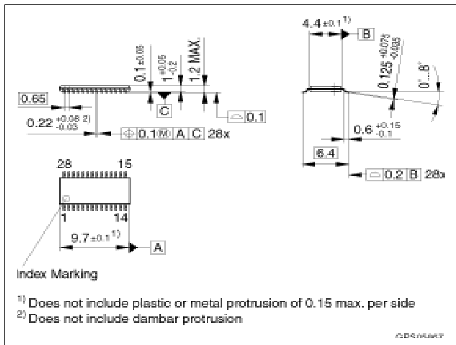
图 18 PG-TSSOP-28-1 封装图
