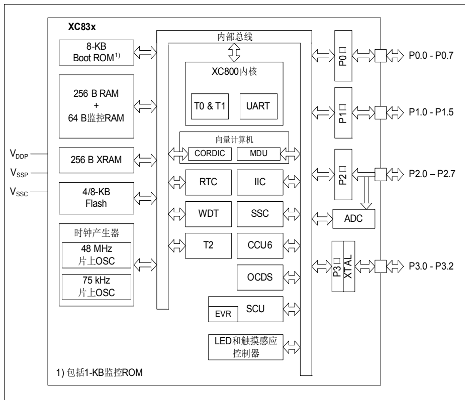
图 2 XC835/836 框图
