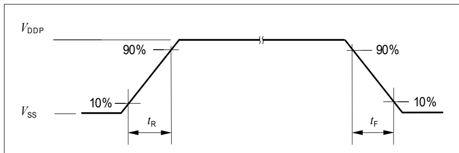
图 11 上升 / 下降时间参数
