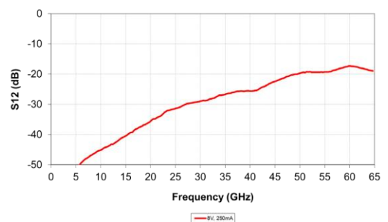
S12
