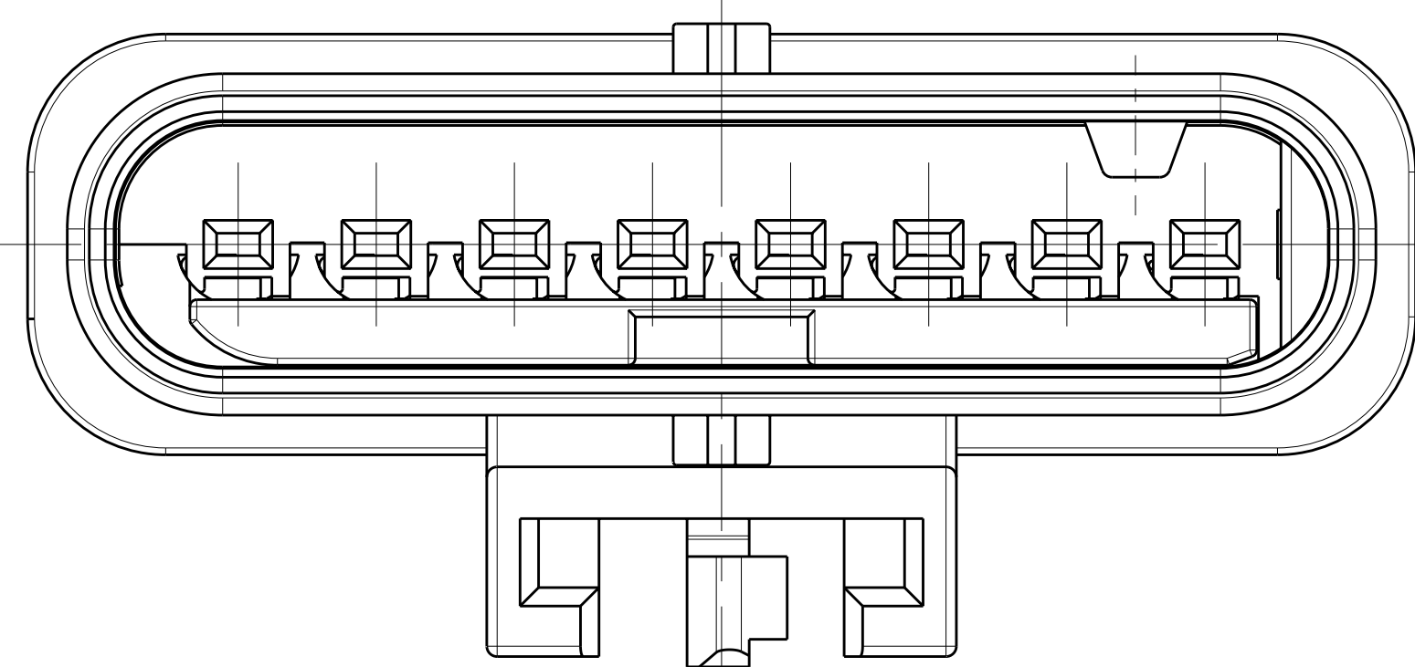
RETAINER IN FINAL LOCKED POSITION 2. Kontaktsicherung in Endraststellung
