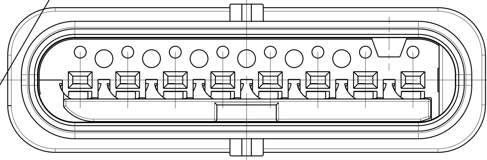
RETAINER IN FINAL LOCKED POSITION 2. Kontaktsicherung in Endraststellung
