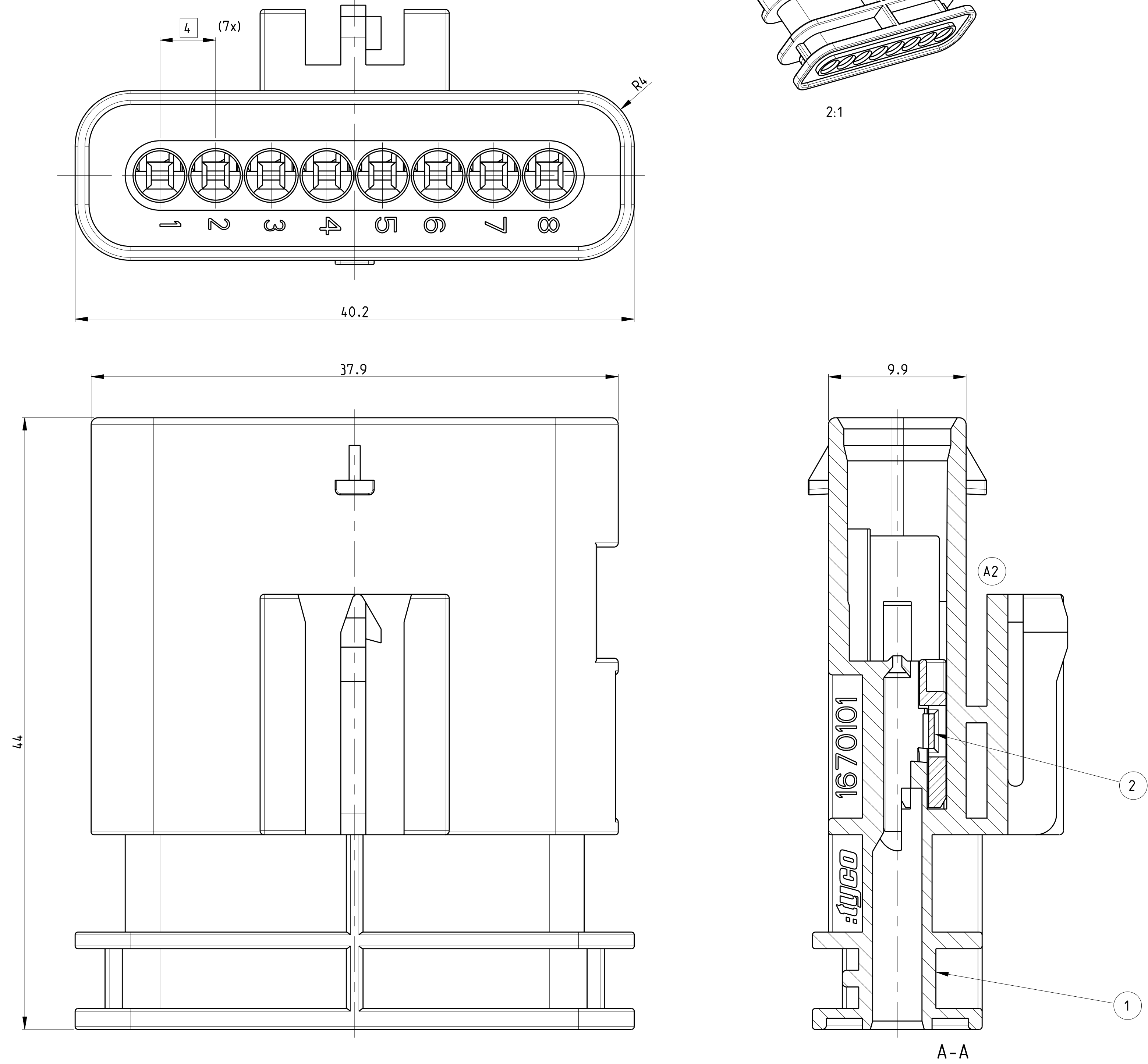
RETAINER IN PRE LOCKED POSITION Kontaktsicherung in Vorraststellung
