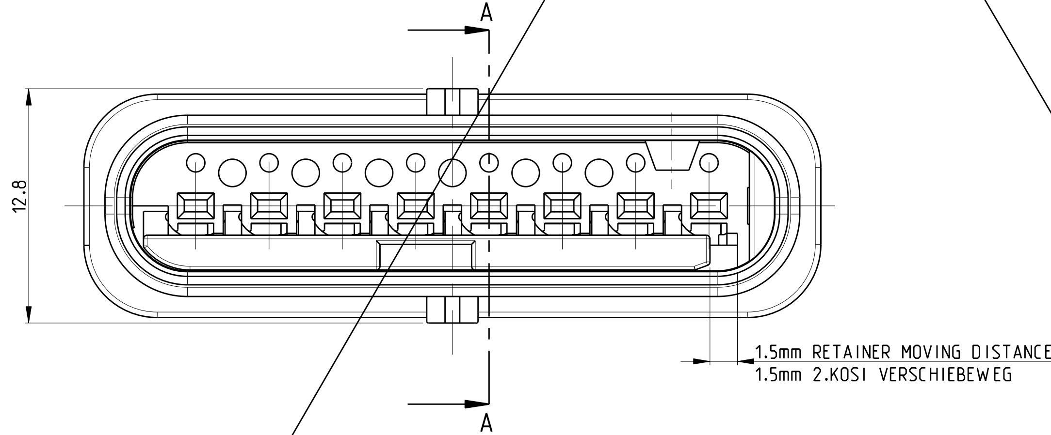
RETAINER IN PRE LOCKED POSITION Kontaktsicherung in Vorraststellung
