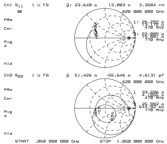
Zin, Zout
