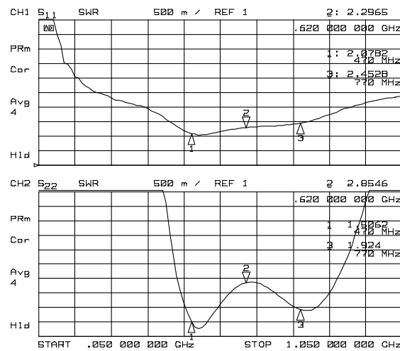
VSWR
