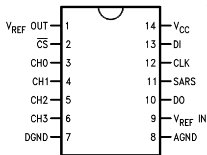
ADC08034
