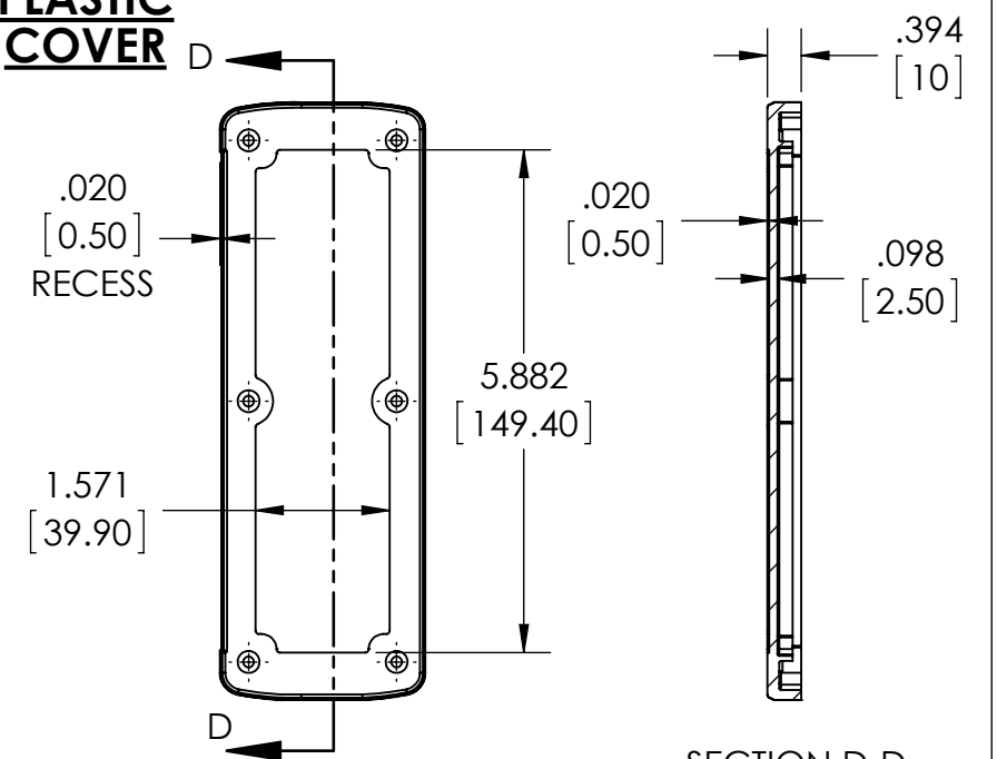
SECTION D-D
