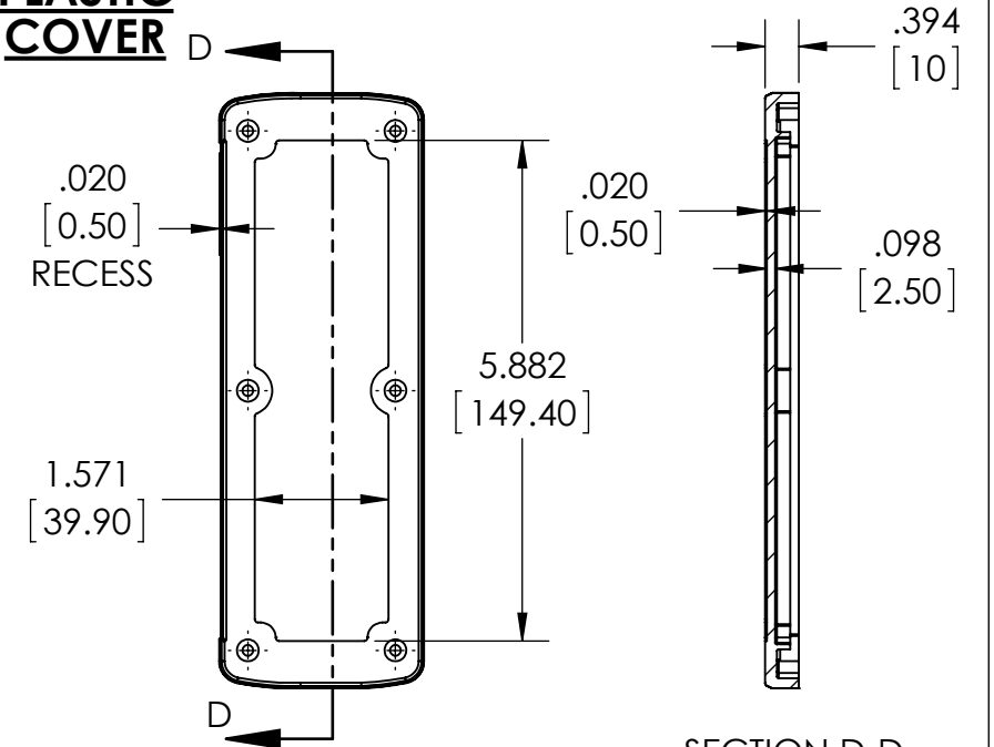
SECTION D-D
