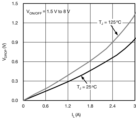
V_{DROP} vs. I_L at V_{IN} = 2.5\text{ V}
