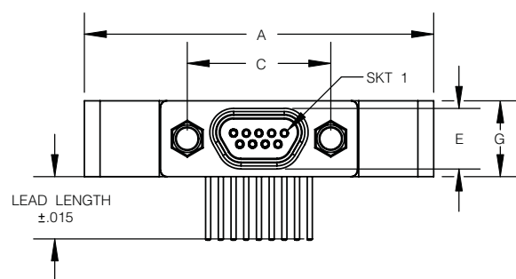
RECEPTACLE
