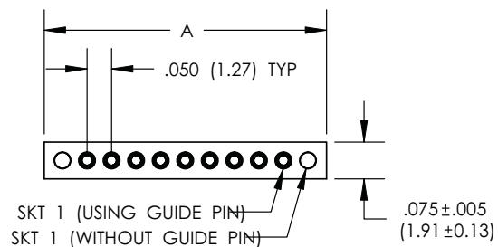
RECEPTACLE
