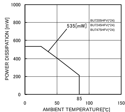
(d) BU7205HFV BU7245HFV BU7475HFV
