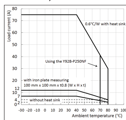
G3NA-275B, G3NA-475B
