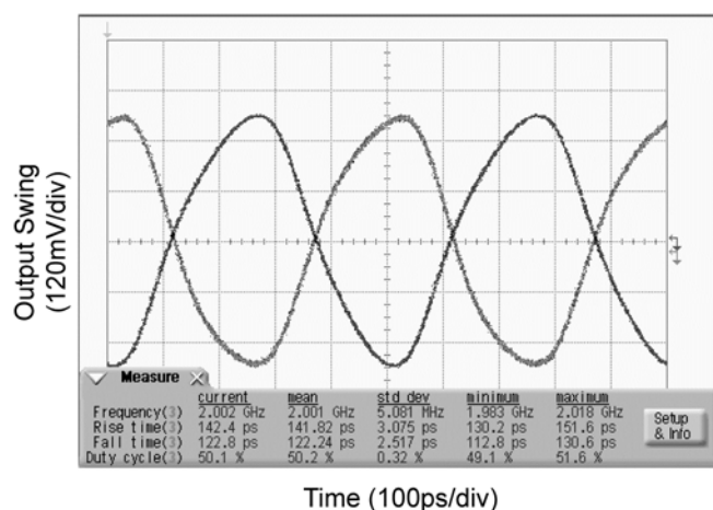
2GHz Output
