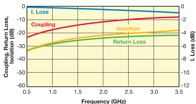
CP0603A****AS
