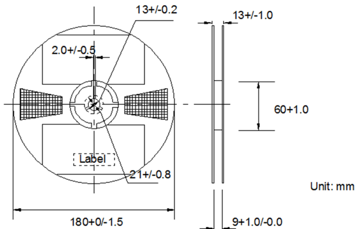
Reel Dimensions
