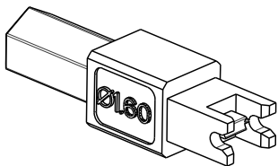
1.6 WIRE (22-24 AWG) 06-9176-7019-02-000 06-9176-7020-02-000
