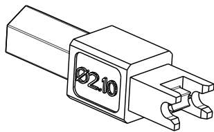
2.1 WIRE (18-20 AWG) 06-9176-7019-01-000 06-9176-7020-01-000
