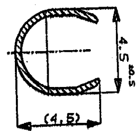
170222 のみ適用 断面 B-B SECT.
