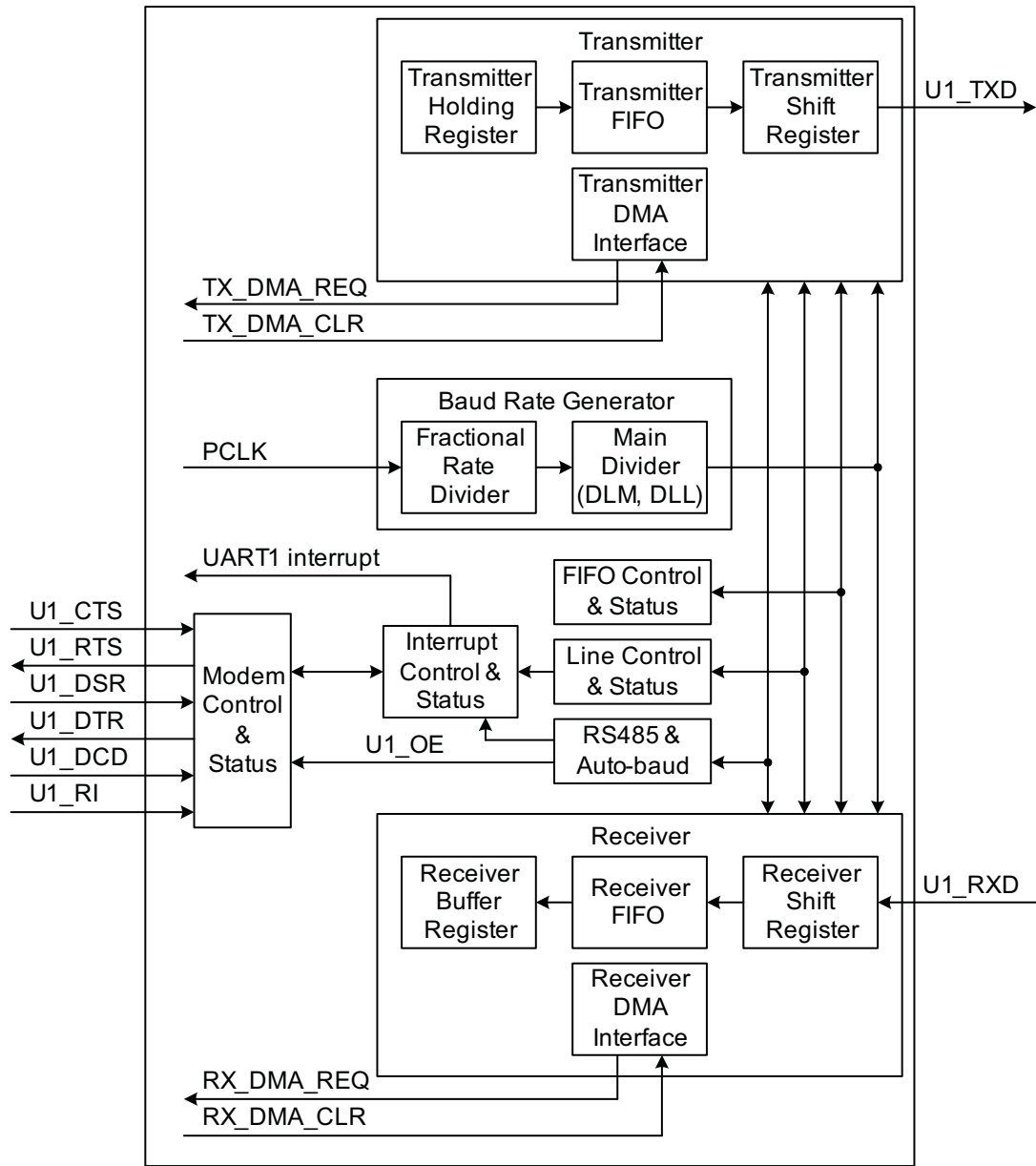
Fig 120.UART1 block diagram
