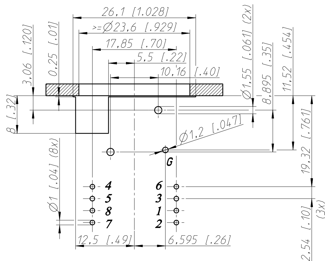
PCB-Layout (component side) Print Bohrplan (Bestueckungsseite)
