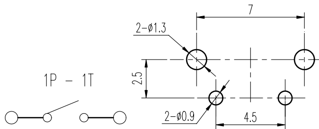
示意图 SCHEMATIC
