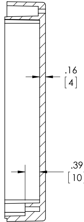
SECTION A-A
