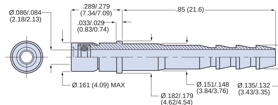
857-010 Socket Contact
