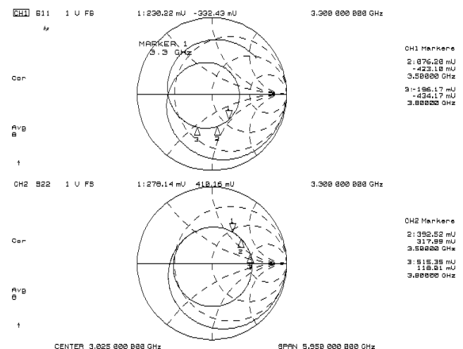
Zin, Zout
