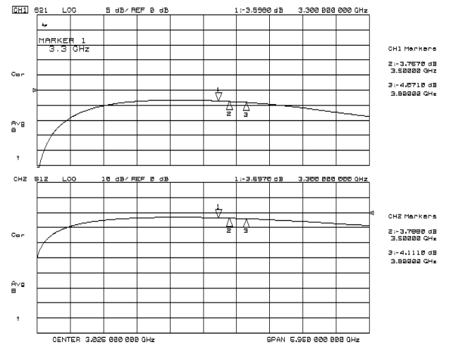
S21, S12
