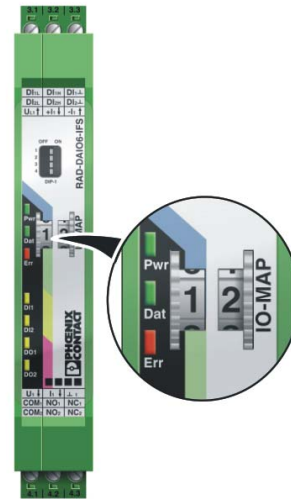
Bild 4 Thumb wheel
