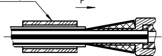
FERRULE
