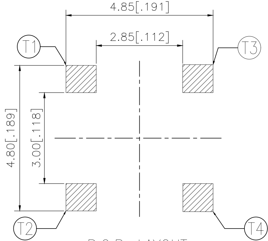
P.C.B. LAYOUT
