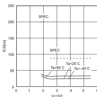
Fig.20 \overline{CS} high time t_{CS}
