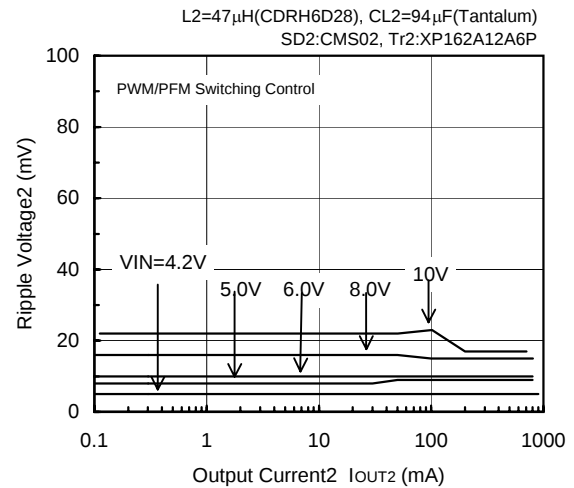
FOSC=180kHz, VOUT2=5.0V
