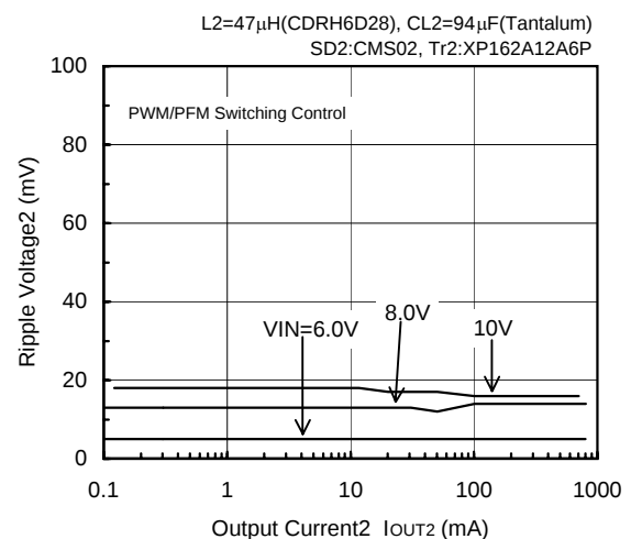
FOSC=180kHz, VOUT2=5.0V
