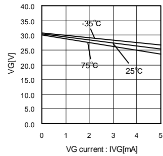
Fig. 3 VG Voltage (BD6761FS)
