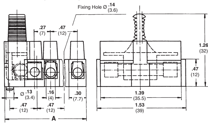
1003Si (2-5 Circuits)
