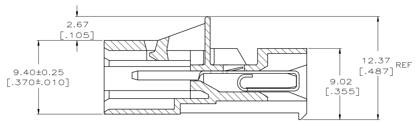
SECTION A-A
