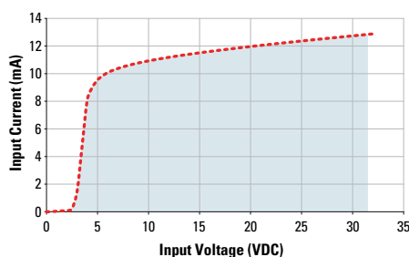
4-32 VDC Input
