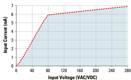
90-280 VAC/VDC Input
