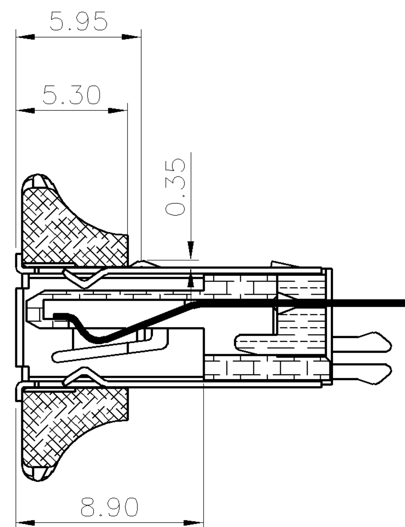
SECTION A-A
