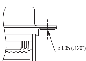
Standard rivet \varnothing 3.05\text{mm} no digit
