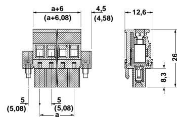
MVSTBW 2,5 HC/...-STF(-5,08)
