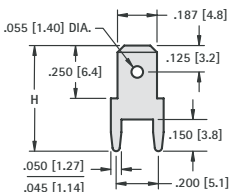
.187 (4.8) TAB
