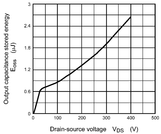
Fig. 8.10 E oss - V DS
