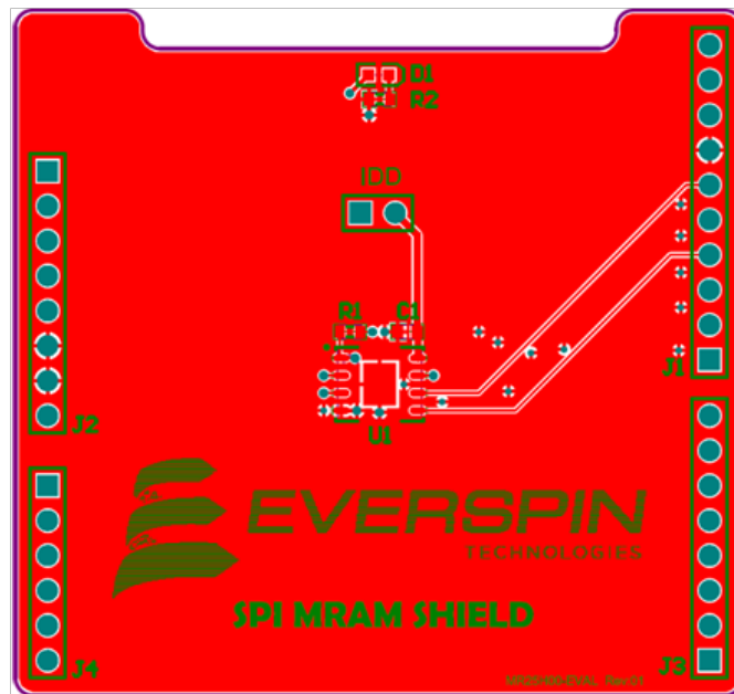
PCB Top
