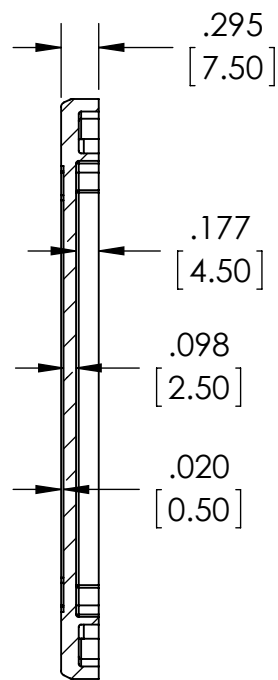
SECTION D-D
